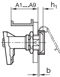
Защелки GN 119
